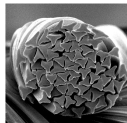
糸の断面写真
